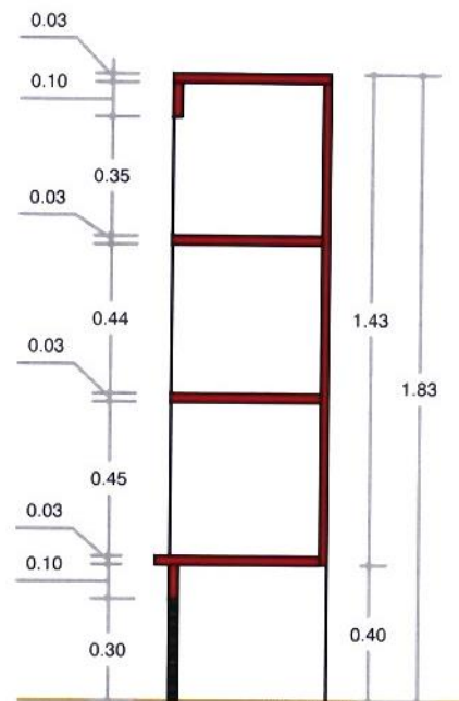
Sección A-A'
