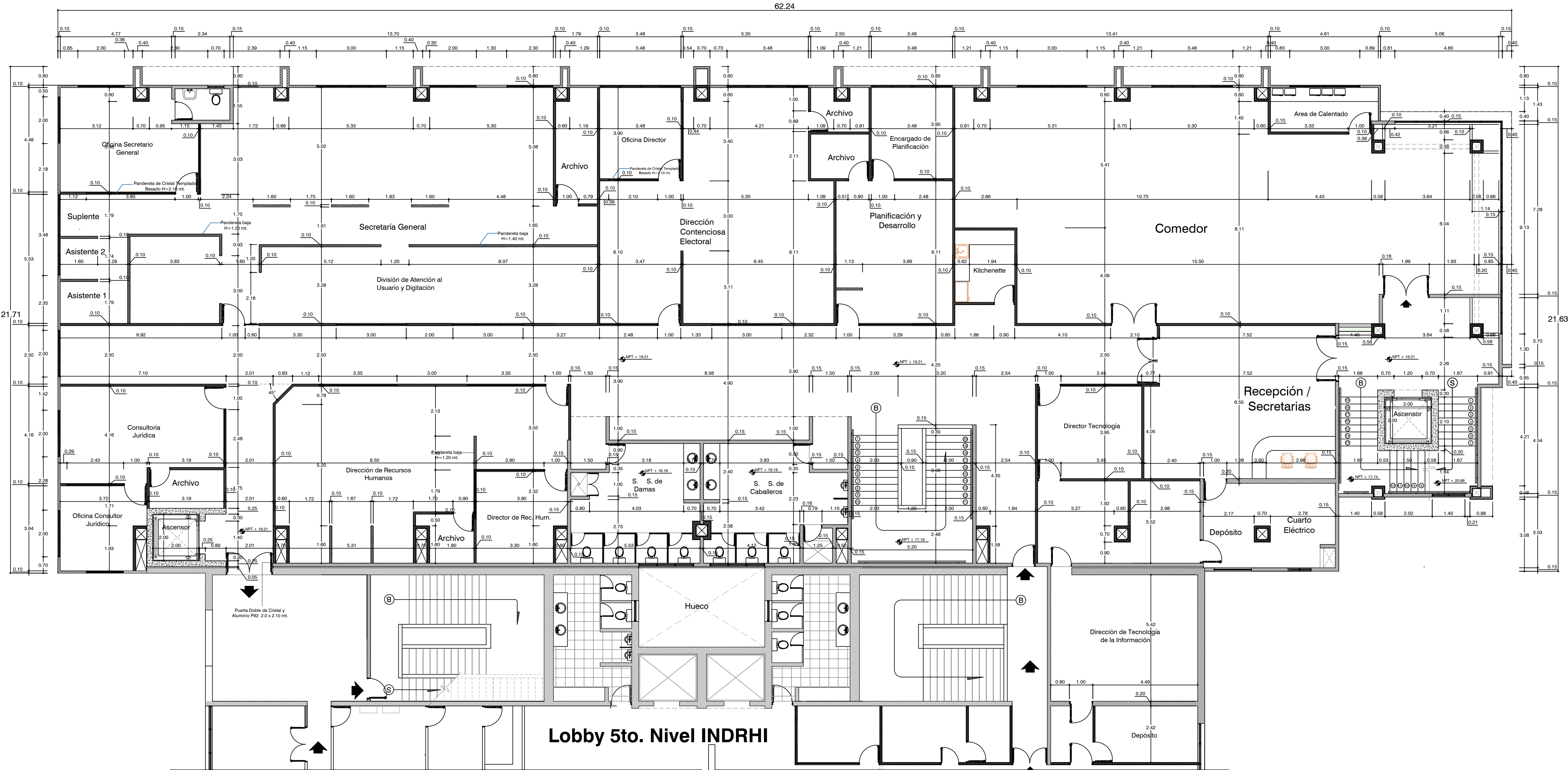
PLANTA DIMENSIONADA PROPUESTA 5TO. NIVEL
