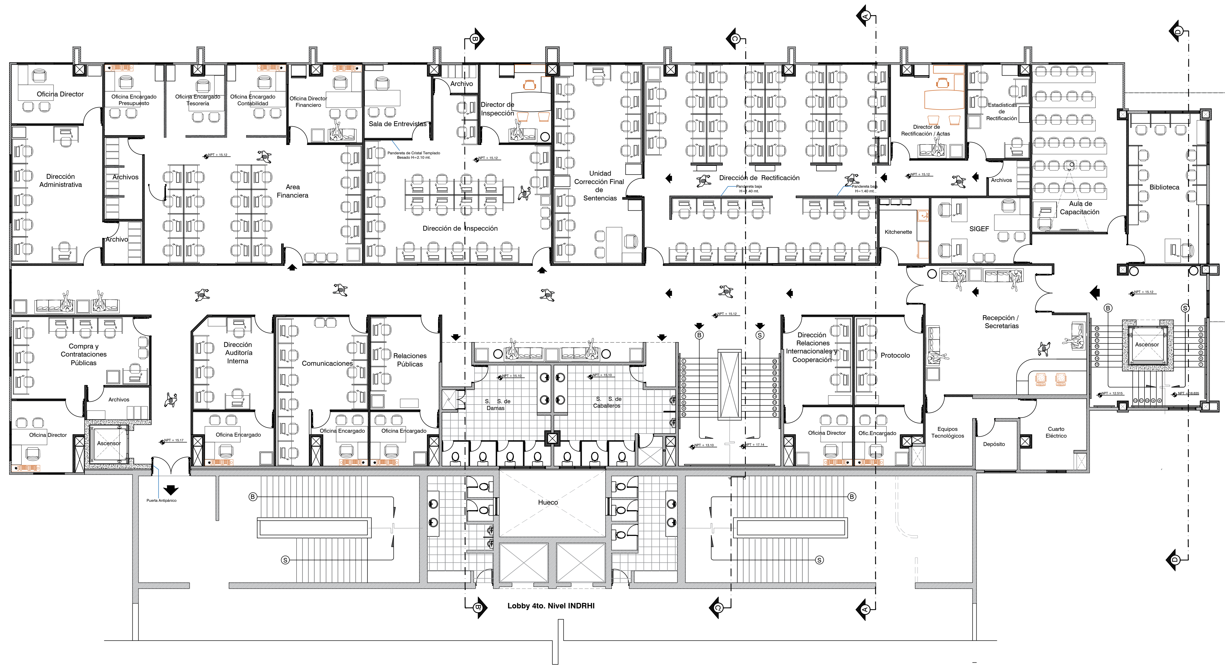
PLANTA ARQUITECTONICA PROPUESTA 4TO. NIVEL
