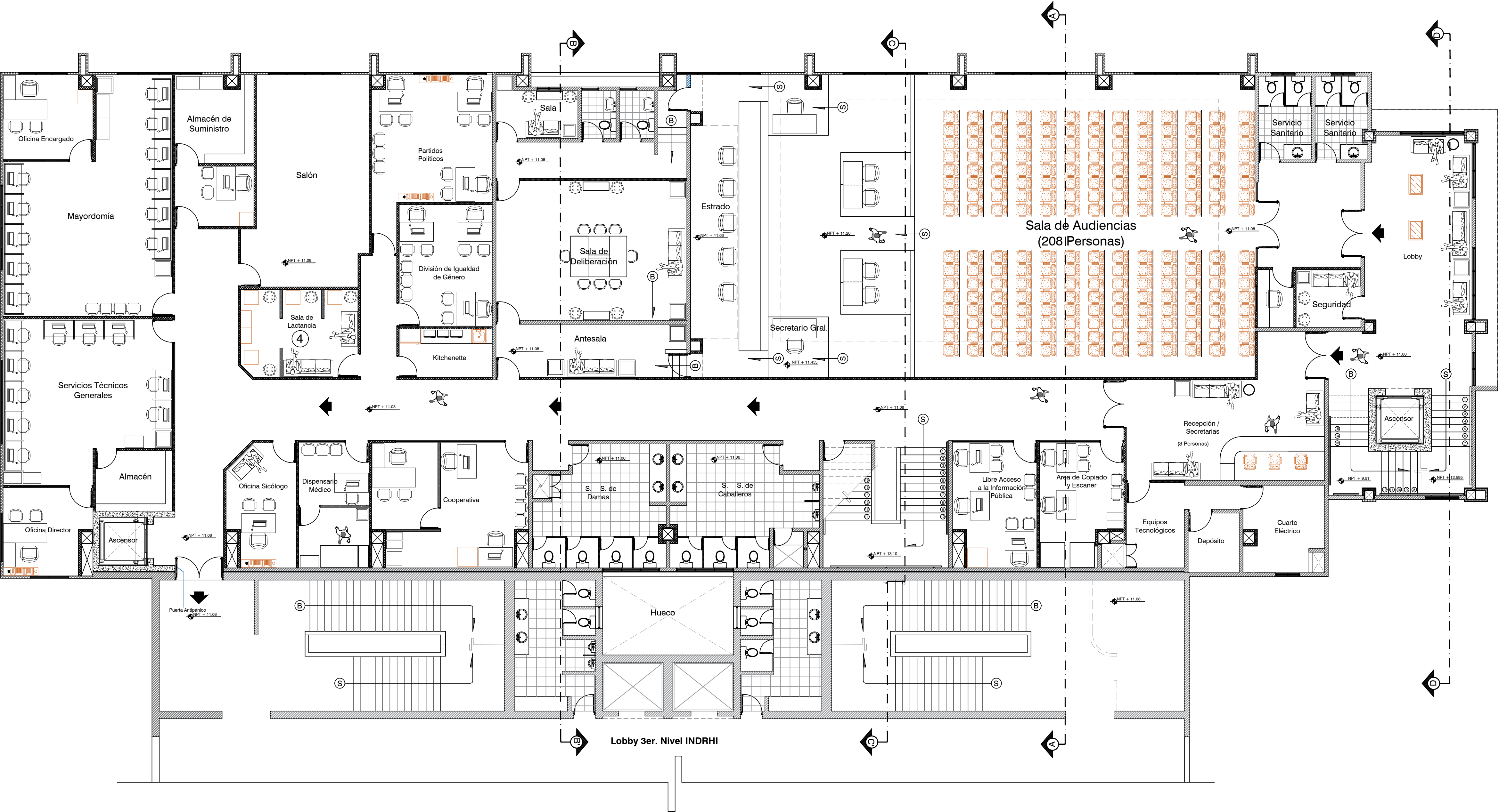
PLANTA ARQUITECTONICA PROPUESTA 3ER. NIVEL
