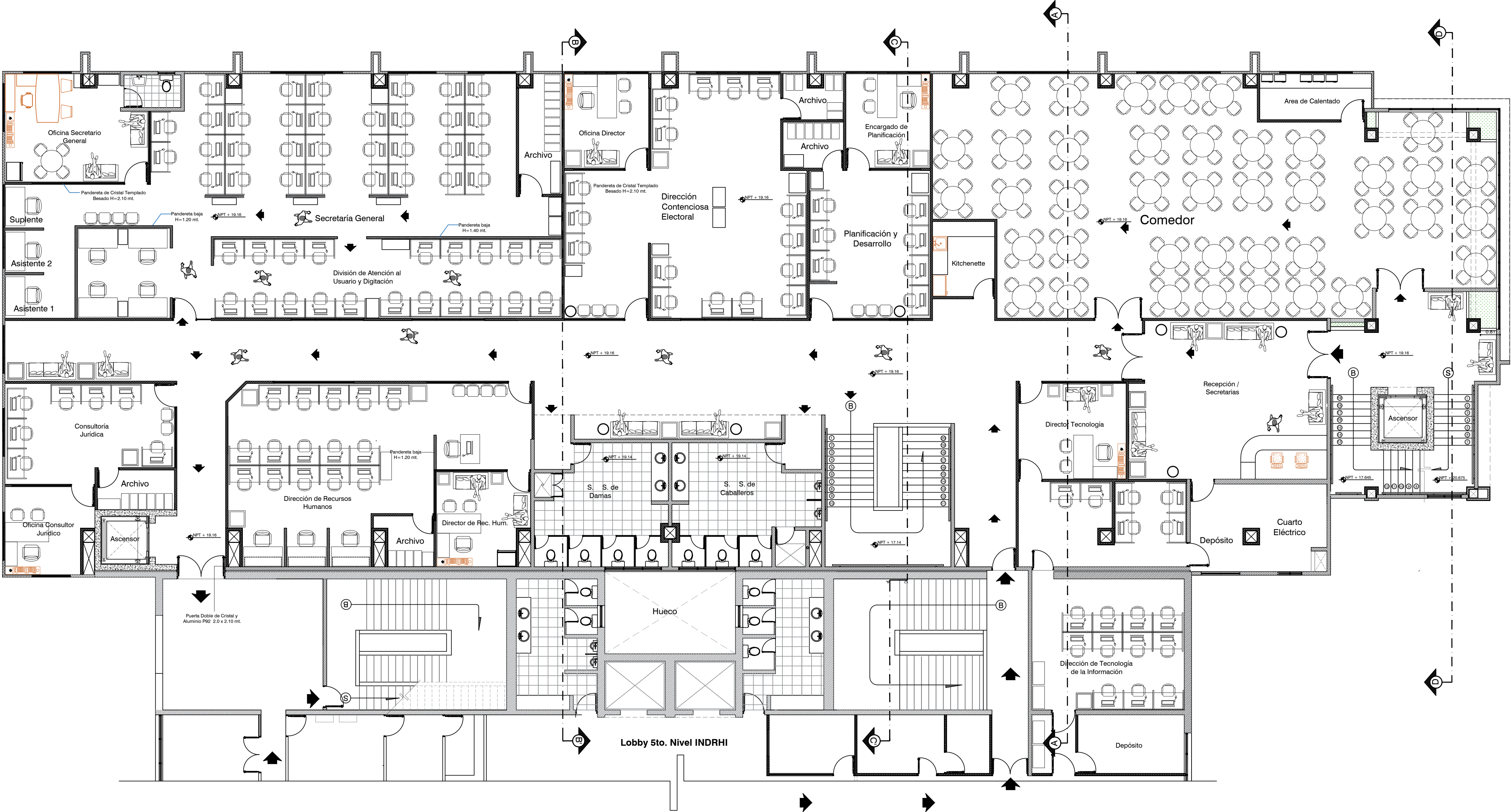
PLANTA ARQUITECTONICA PROPUESTA 5TO. NIVEL TSE
