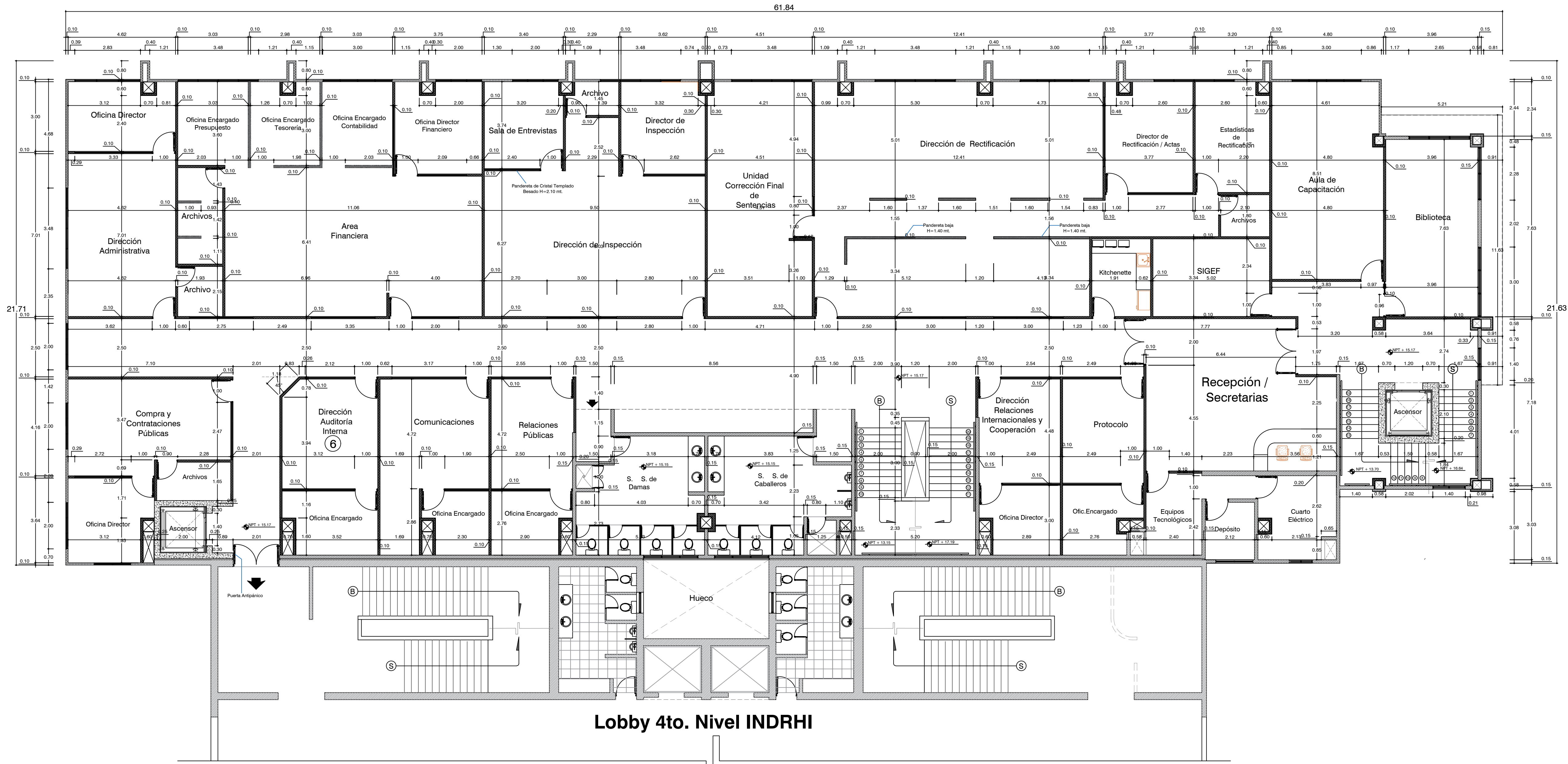
PLANTA DIMENSIONADA PROPUESTA 4TO. NIVEL
